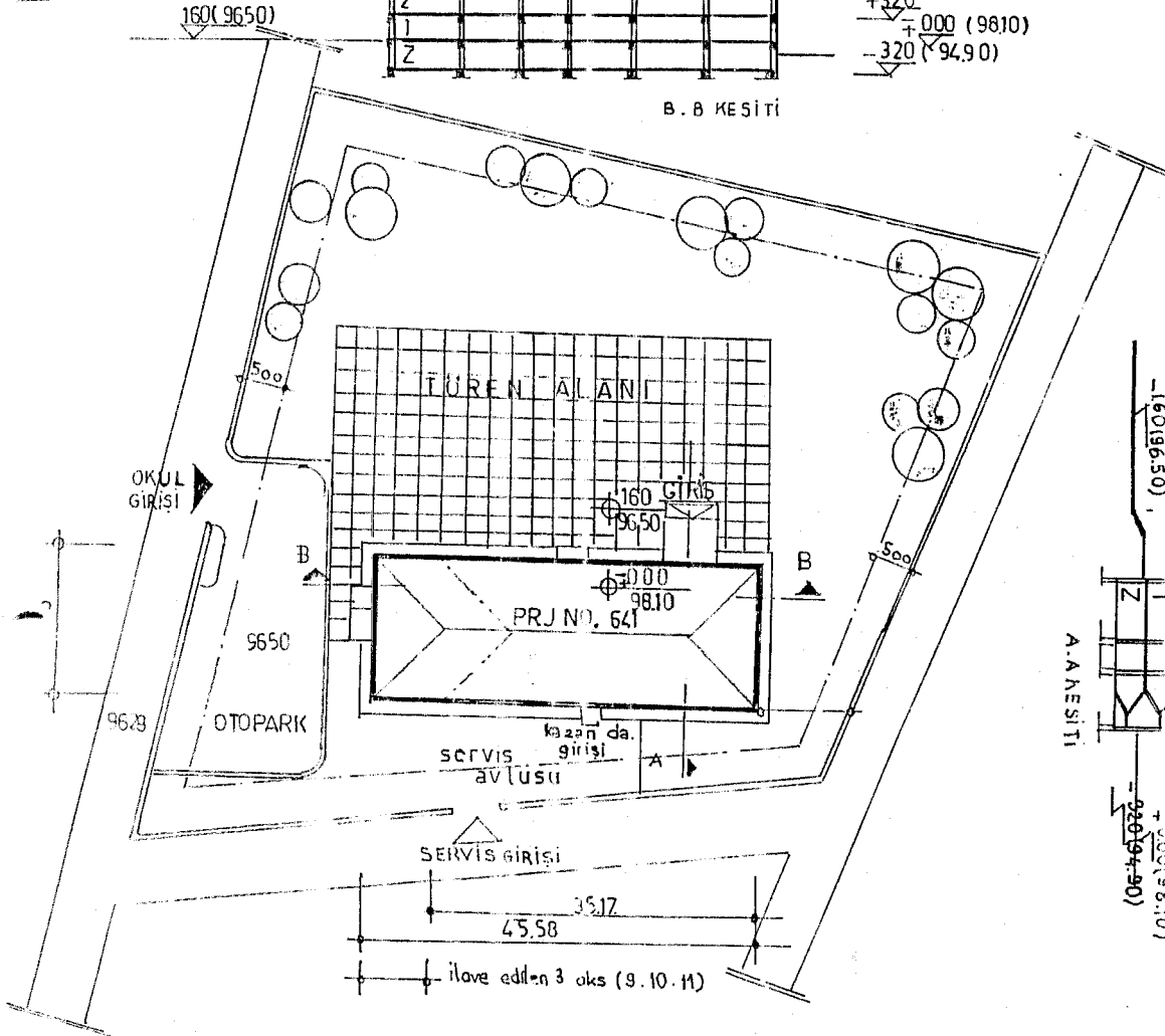
vaziyet planı
