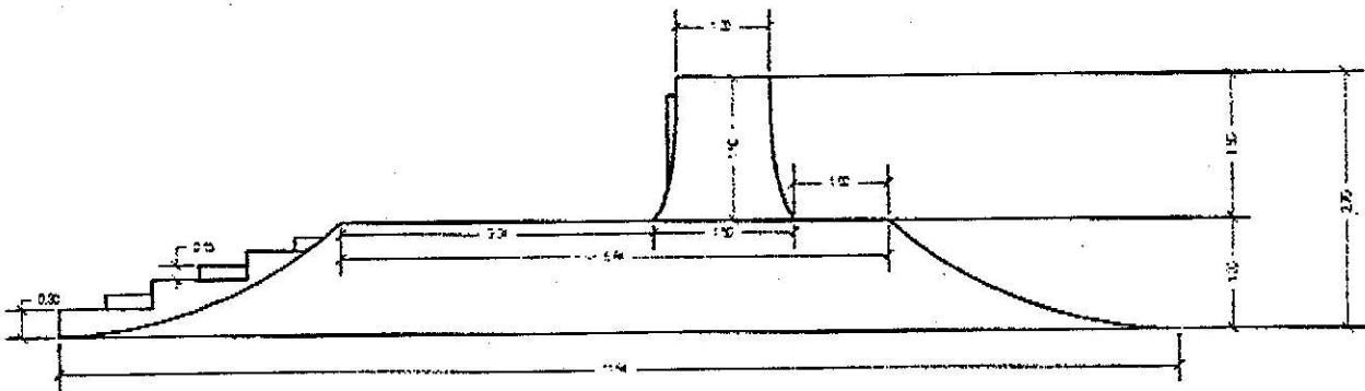
SAĞ YAN GÖRÜNÜŞ
