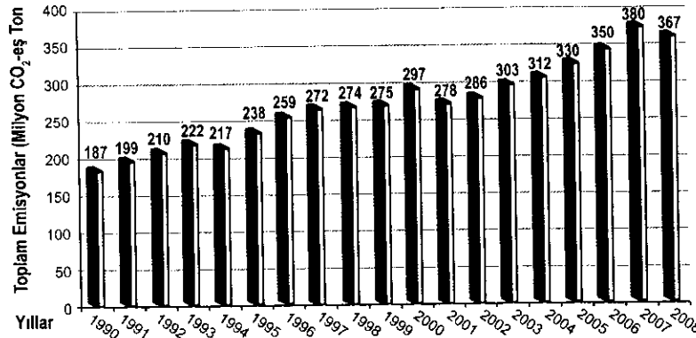
Şekil 9 - Yıllar itibarıyla Türkiye'nin Kümülatif Sera Gazı Emisyonlarının Gelişimi
