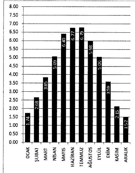
AĞRI İLİ GLOBAL RADYASYON DEĞERLERİ (KWh/m 2 -gün)
