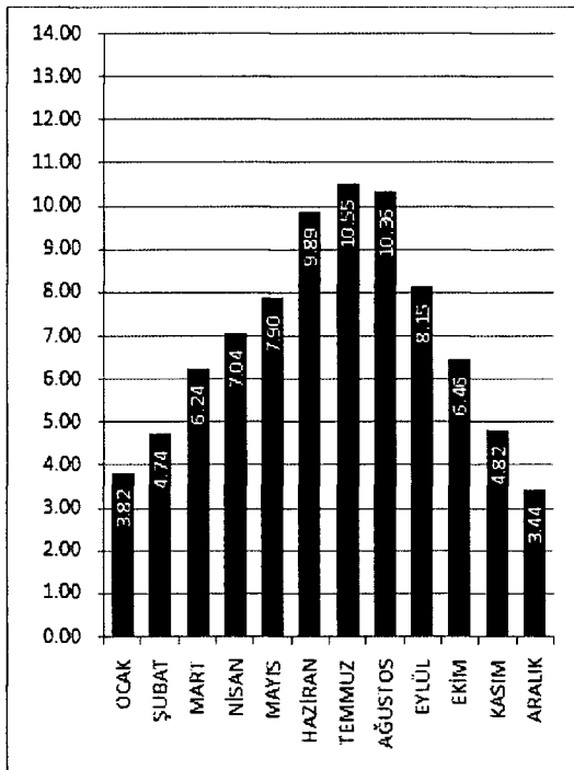
KARS İLİ GÜNEŞLENME SÜRESİ DEĞERLERİ (Saat)
