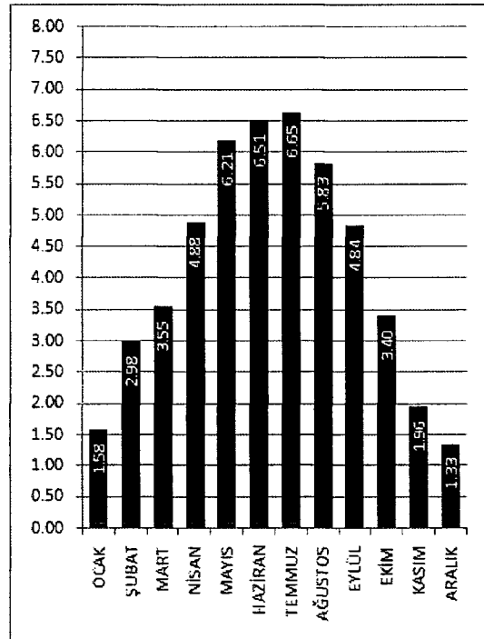
KARS İLİ GLOBAL RADYASYON DEĞERLERİ (KWh/m²-gün)
