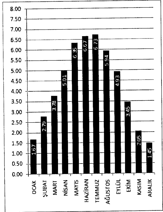
ERZURUM İLİ GLOBAL RADYASYON DEĞERLERİ (KWh/m 2 -gün)
