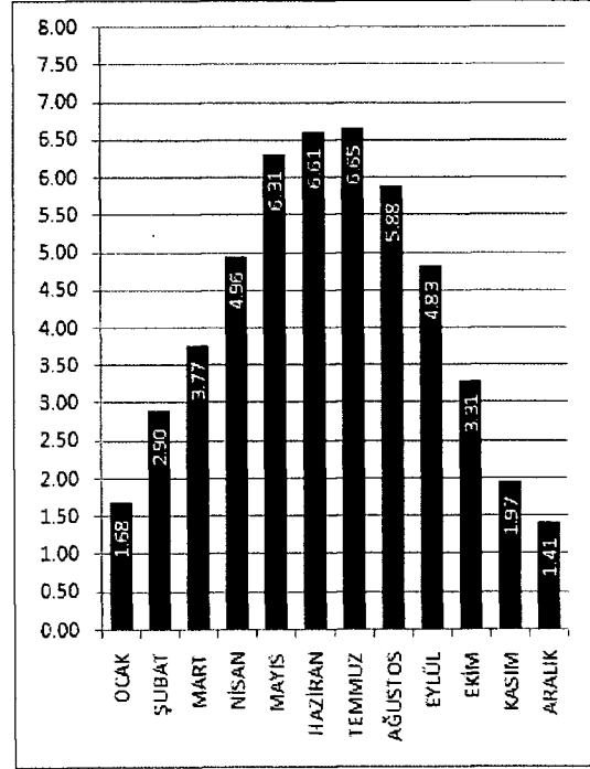
BAYBURT İLİ GLOBAL RADYASYON DEĞERLERİ (KWh/m 2 -gün)
