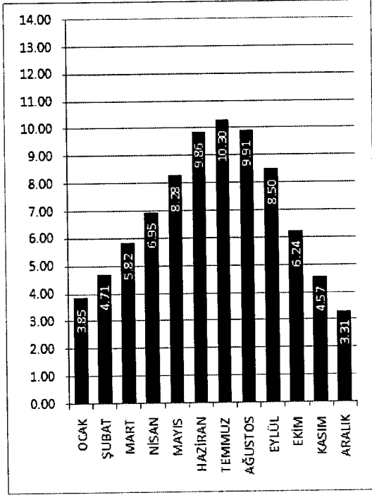
ERZURUM İLİ GÜNEŞLENME SÜRESİ DEĞERLERİ (Saat)
