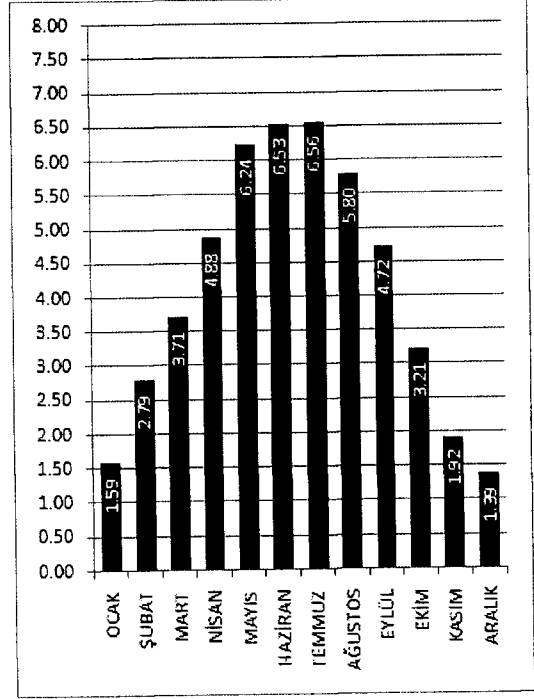
GÜMÜŞHANE İLİ GLOBAL RADYASYON DEĞERLERİ (KWh/m 2 -gün)
