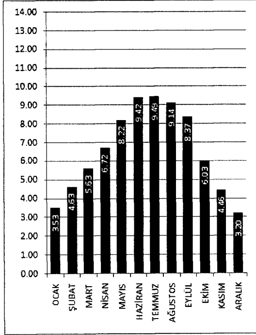
BAYBURT İLİ GÜNEŞLENME SÜRESİ DEĞERLERİ (Saat)
