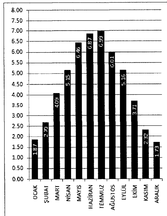
BİTLİS İLİ GLOBAL RADYASYON DEĞERLERİ (KWh/m²-gün)
