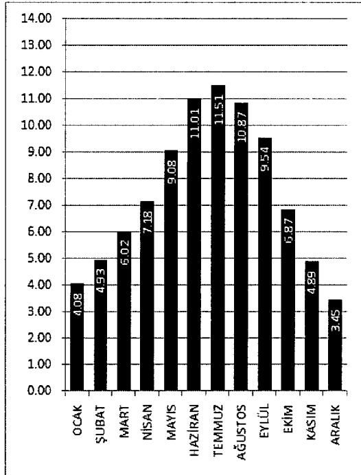
BİNGÖL İLİ GÜNEŞLENME SÜRESİ DEĞERLERİ (Saat)
