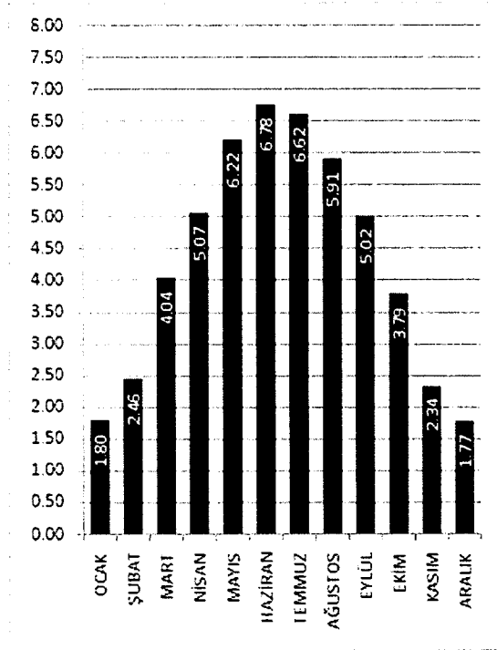
BATMAN İLİ GLOBAL RADYASYON DEĞERLERİ (KWh/m 2 -gün)
