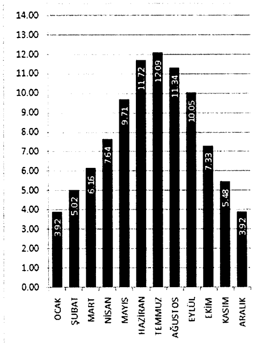
BATMAN İLİ GÜNEŞLENME SÜRESİ DEĞERLERİ (Saat)
