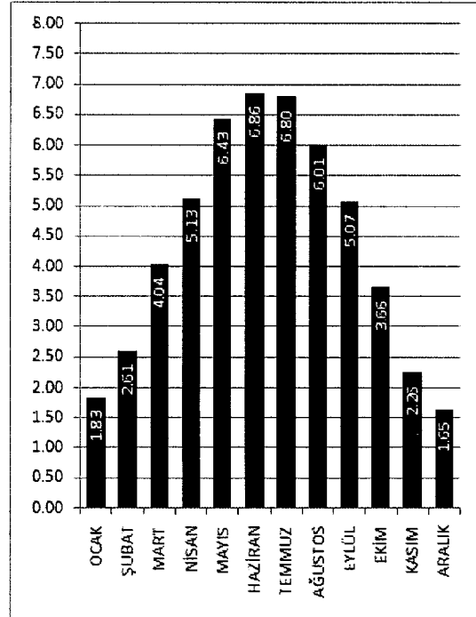
BİNGÖL İLİ GLOBAL RADYASYON DEĞERLERİ (KWh/m²-gün)
