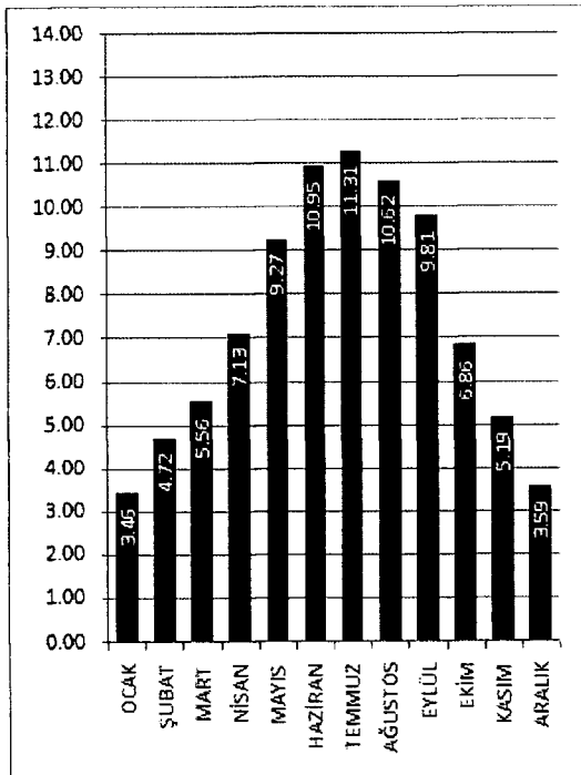
BİTLİS İLİ GÜNEŞLENME SÜRESİ DEĞERLERİ (Saat)
